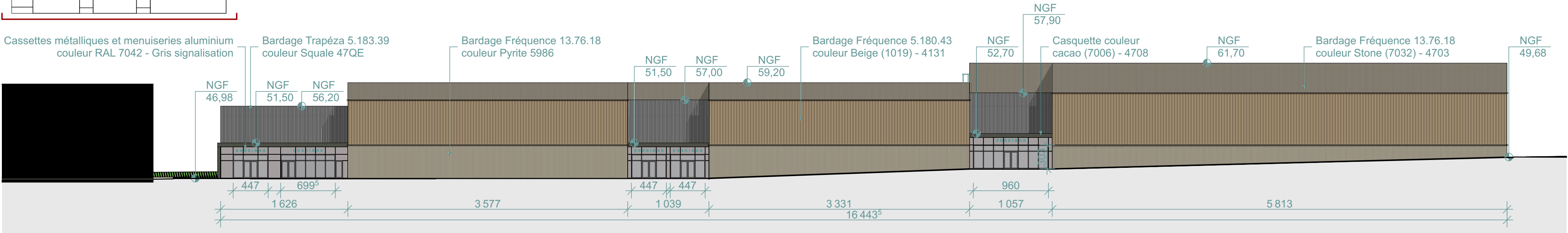
FAÇADE SUD
