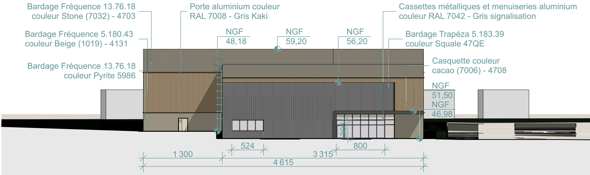
FAÇADE OUEST
